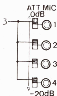
Figure 2-3 MIC ATT
