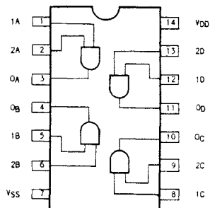
IC-20 IMC 14081 (MC 14081B)
